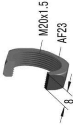
Przeciwnakrętka KM20
