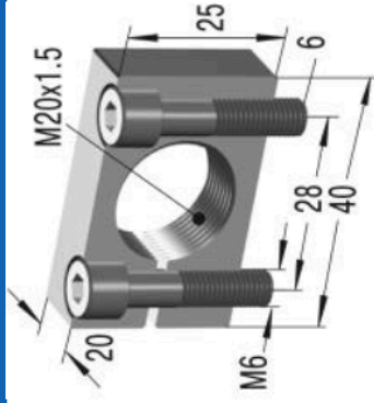
Kołnierz zaciskowy MB20
