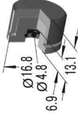
Głowica stalowo-polimerowa BP20
