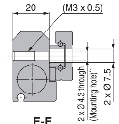
E-E
