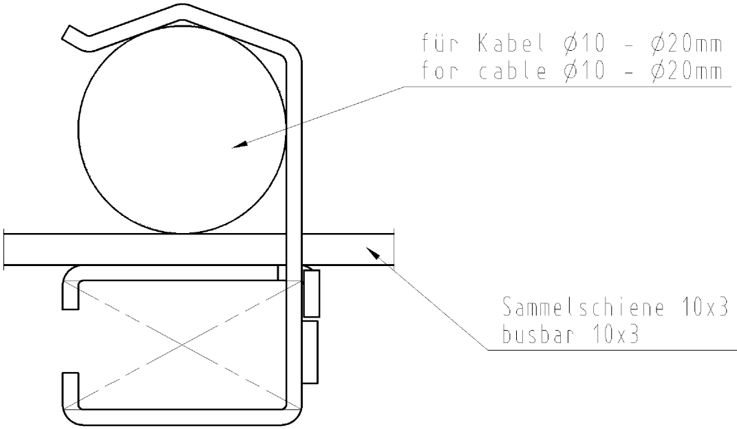
montierter Zustand/mounted state M 2:1
