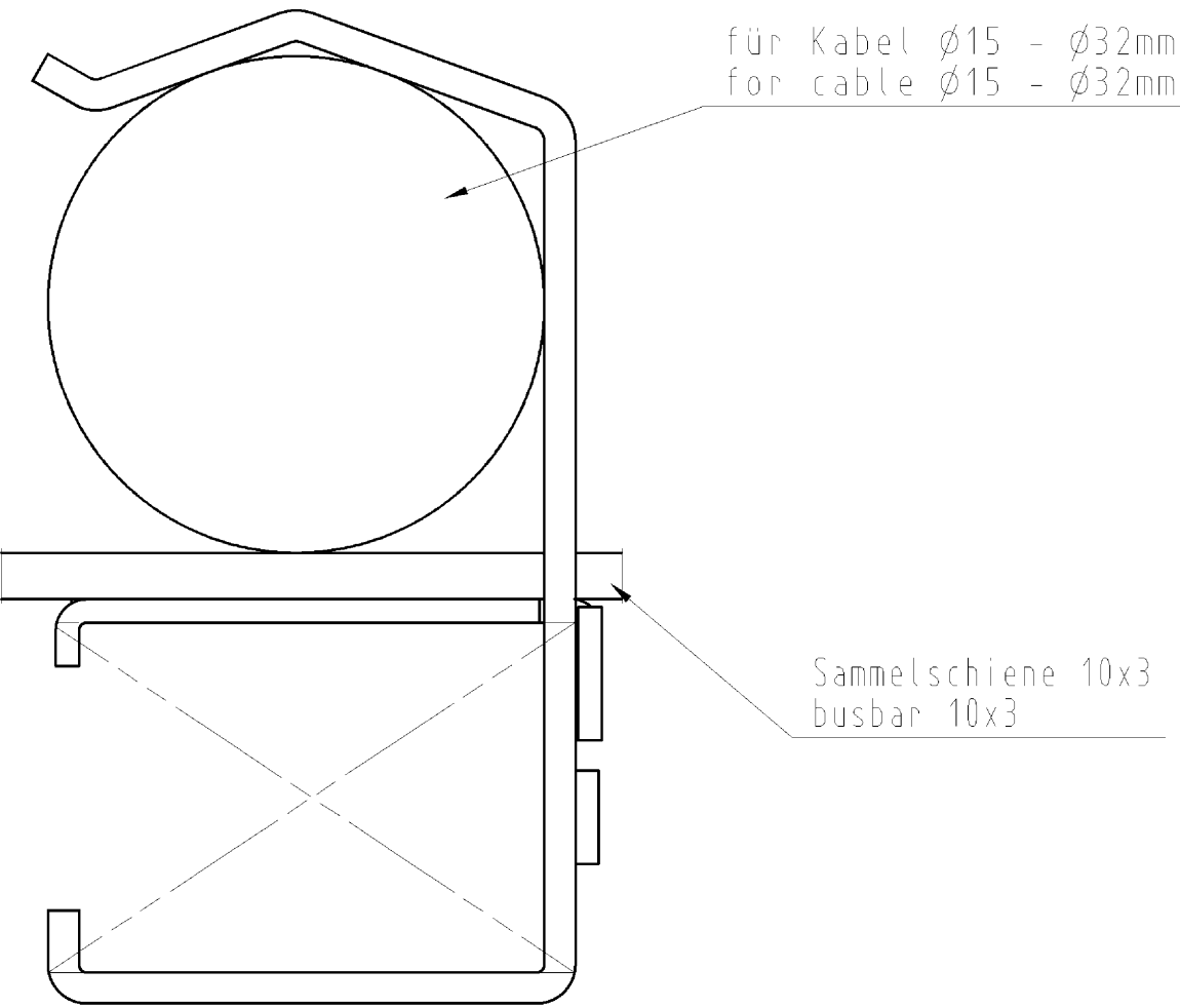
montierter Zustand/mounted state M 2:1
