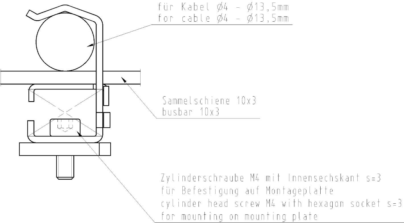
montierter Zustand/mounted state M 2:1
